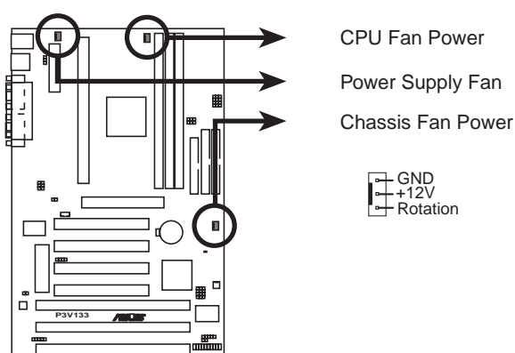
P3V133 12Volt Cooling Fan Power
