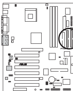
P4B-E IDE Connectors
