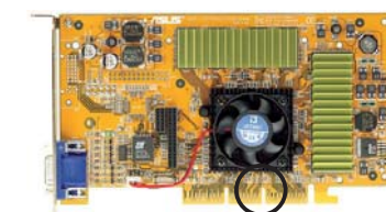
Keyed for 1.5v 使用 1.5V 電壓的 AGP 卡特徵
