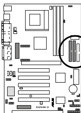
CUV4X-V IDE Connectors
