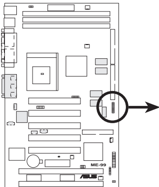
ME-99 LCD Header
