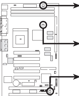
ME-99 12-Volt Cooling Fan Power
