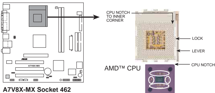
A7V8X-MX Socket 462
