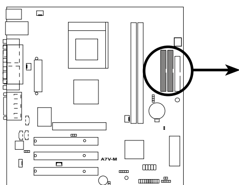
A7V-M IDE Connectors
