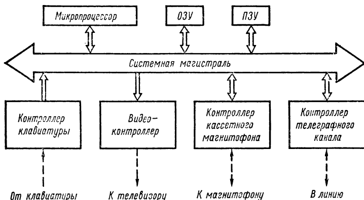
Рис. 6.2. Функциональная схема микроЭВМ
