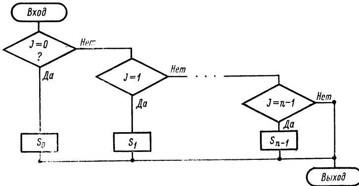
Рис. 4.8. Блок-схема структуры варианта
