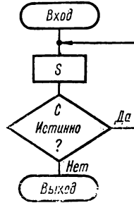
Рис. 4.7. Блок-схема структуры цикла с постусловием
