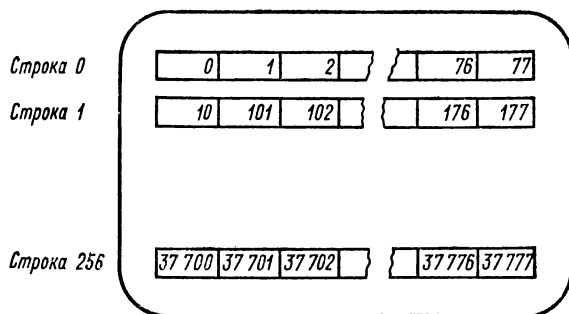
Рис. 6.12. Расположение байтов растровой памяти на экране
