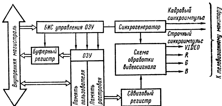
Рис. 6.11. Структурная схема формирования выходных телевизионных сигналов
