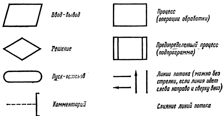
Рис. 4.2. Стандартные символы блок-схемы
