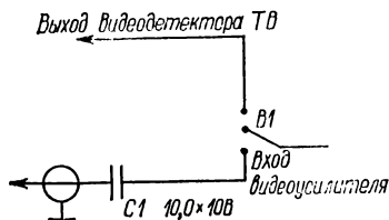
Рис. 6.9. Схема организации видеовхода
