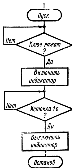
Рис. 4.3. Блок-схема системы «ключ — индикатор»
