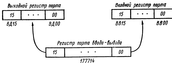
Рис. 6.7. Работа с портом ввода—вывода
