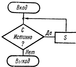
Рис. 4.6. Блок-схема структуры цикла с предусловием
