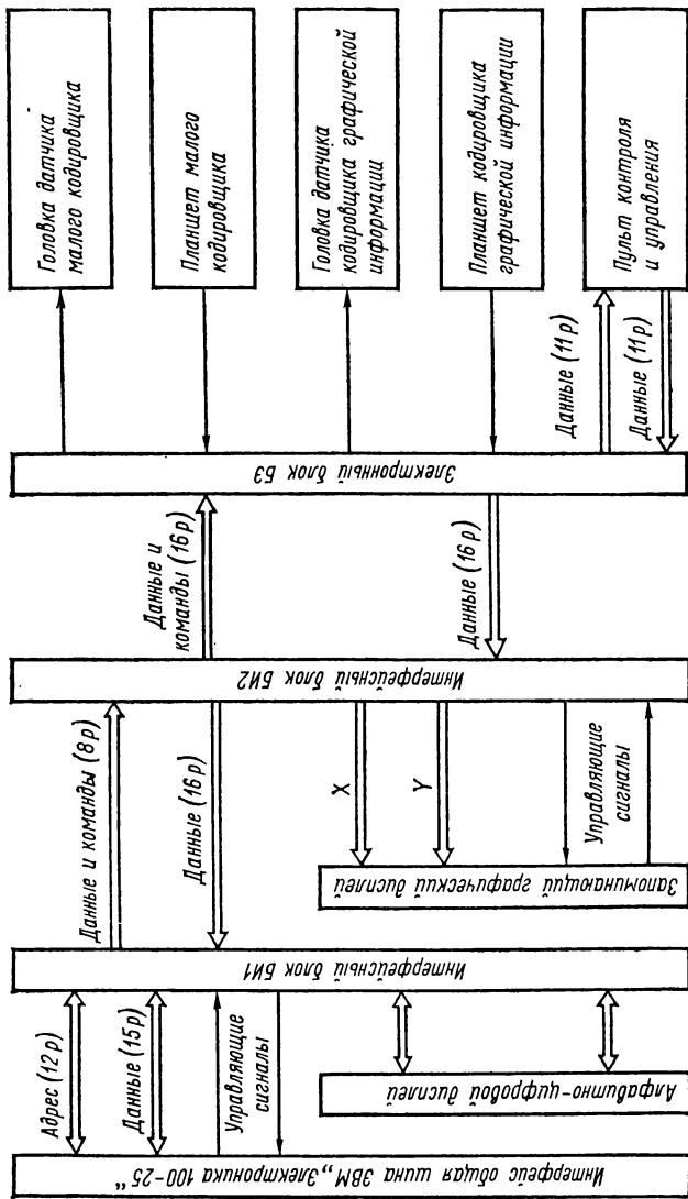
Рис. 7.4. Упрощенная структурная схема подсистемы отображения и диалога
