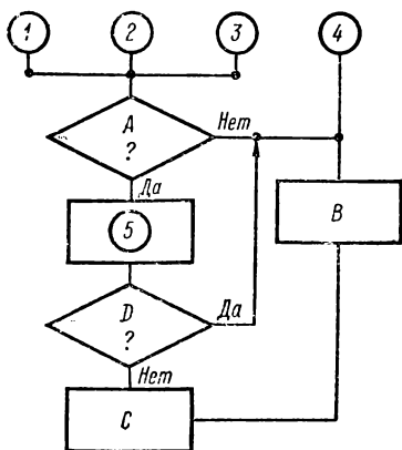
Рис. 4.4. Блок-схема неструктурированной программы
