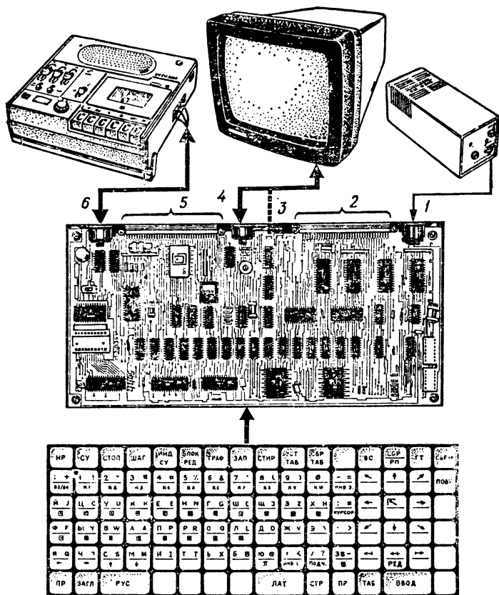
Рис. 6.1. Структурная схема БК: 1 — разъем для подключения блока питания; 2 — разъем порта ввода-вывода; 3 — разъем для подключения цветного телевизора; 4 — разъем для подключения черно-белого телевизора; 5 — разъем системной магистрали микроЭВМ; 6 — разъем для подключения магнитофона
