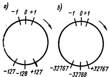
Рис. 3.1. Диаграмма изменения значений индексов. — для переменных с одним индексом
