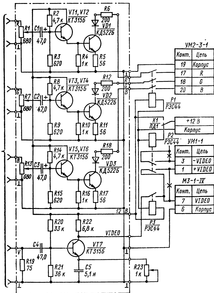
Рис. 6.10. Принципиальная схема согласующей платы
