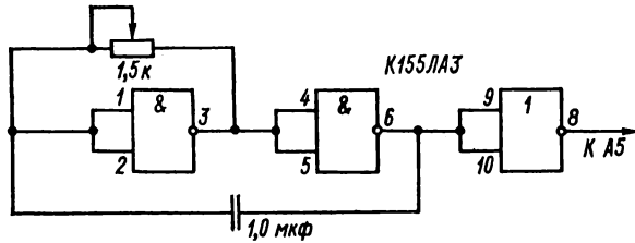
Рис. 3.4. Схема генератора импульсов
