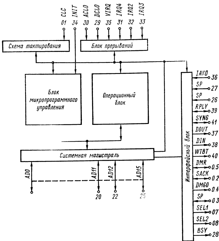
Рис. 6.3. Структурная организация микропроцессора K1801BM1
