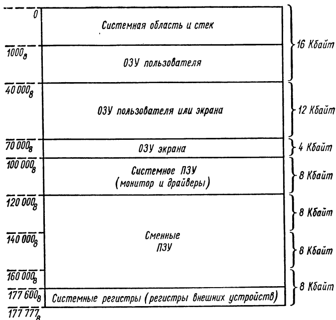
Рис. 6.4. Распределение адресного пространства микроЭВМ
