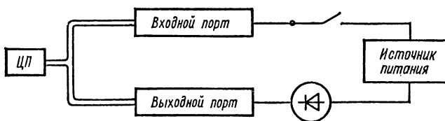
Рис. 4.1. Система «ключ—индикатор»
