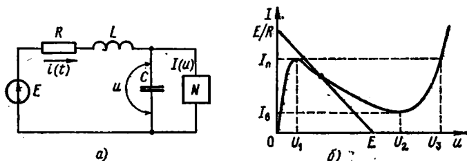
Рис. 7.13. Цепь с нелинейным элементом (а) и его N -образная вольт-амперная характеристика (б)
