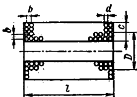
Рис. 7.5. Многослойная короткая цилиндрическая катушка
