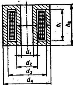
Рис. 7.6. Катушка на броневом сердечнике
