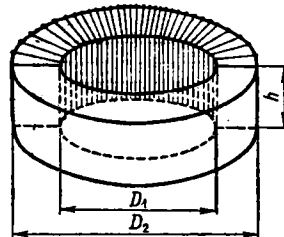
Рис. 7.4. Торoidalная катушка прямоугольного сечения
