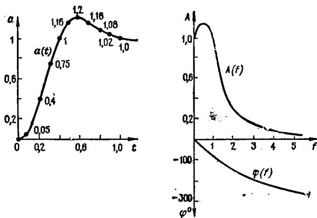
Рис. 5.9. Переходная характеристика (слева) и рассчитанные по ней АЧХ и ФЧХ (справа)
