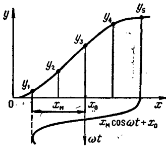
Рис. 5.5. Иллюстрация к методу пяти ординат
