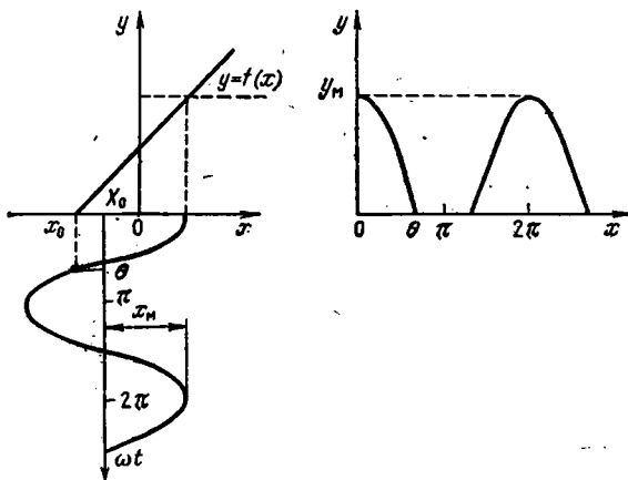
Рис. 5.6. Иллюстрация к методу Берга
