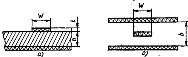
Рис. 7.9. Полосковые несимметричные (а) и симметричные (б) линии
