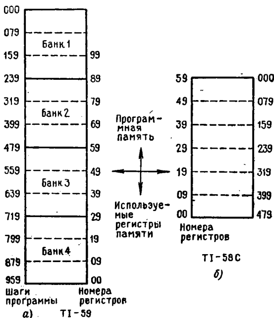
Рис. 2.4. Структура ОЗУ
