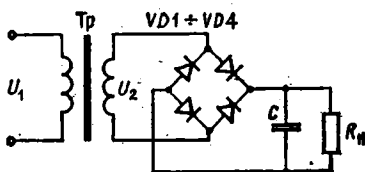
Рис. 7.10. Мостовой выпрямитель
