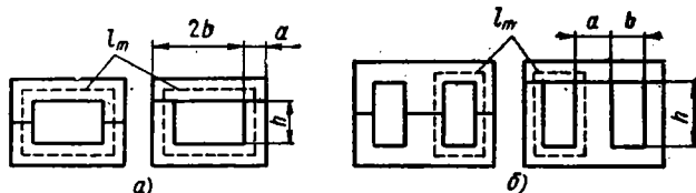
Рис. 7.7. Сердечники из элементов П- (а) и Ш-образной формы (б)
