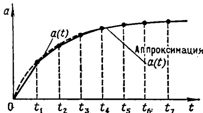
Рис. 5.8. К аппроксимации a(t)
