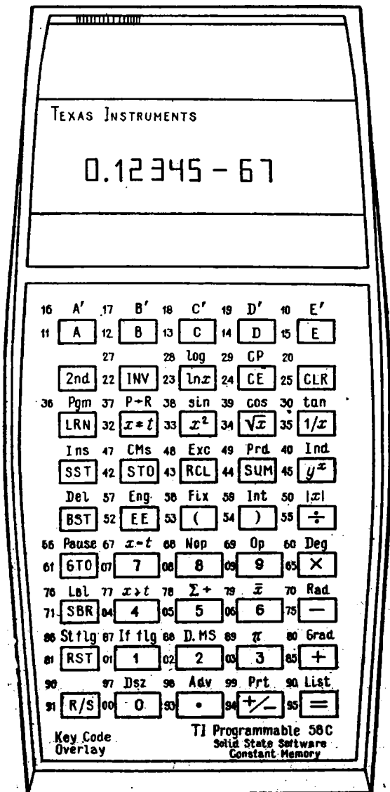
Рис. 2.2. Внешний вид программируемого микрокалькулятора TI-58C с алгебраической логикой вычислений
